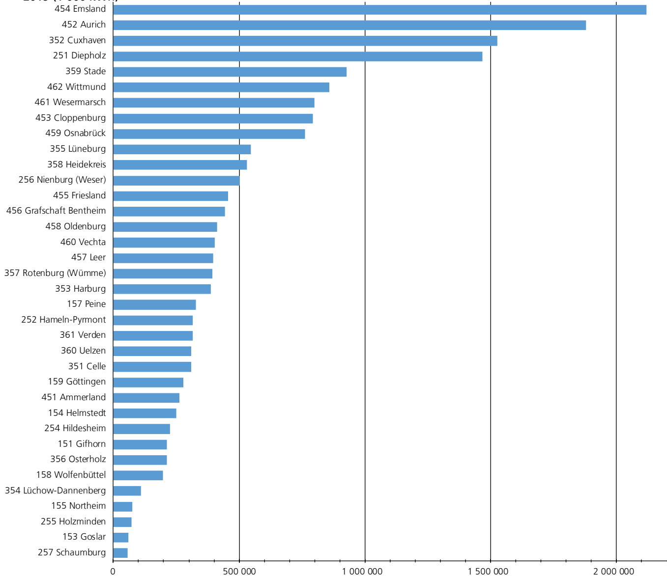
A7 | Nach dem Erneuerbare-Energien-Gesetz (EEG) geförderte Stromeinspeisung aus Windkraft (Land) in den Landkreisen 2019 (1 000 kWh)
