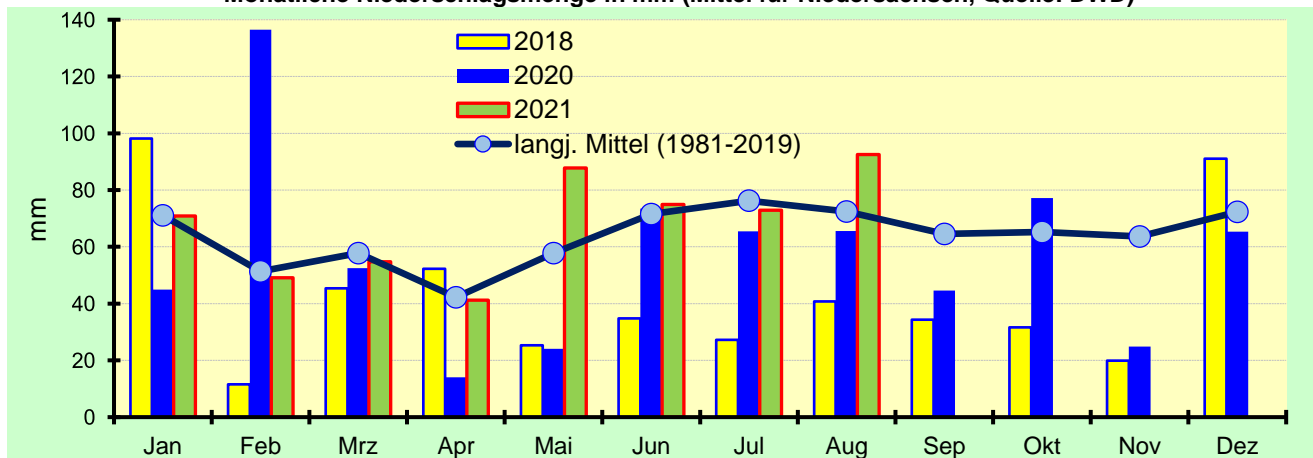
Monatliche Niederschlagsmenge in mm (Mittel für Niedersachsen, Quelle: DWD)
