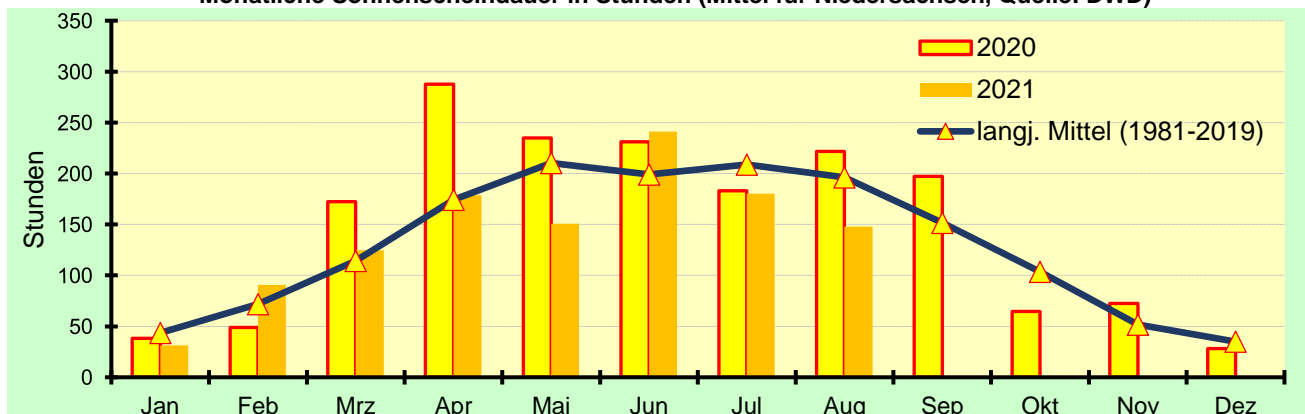
Monatliche Sonnenscheindauer in Stunden (Mittel für Niedersachsen, Quelle: DWD)
